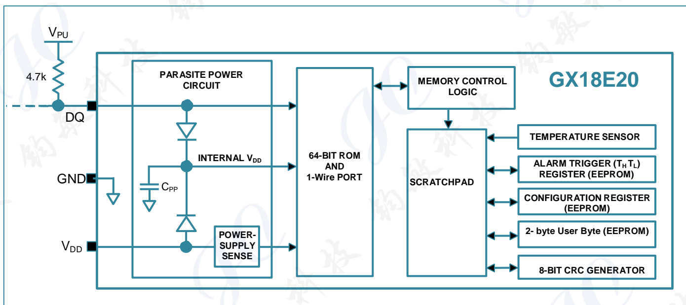
图 1. GX18E20 的结构框图
