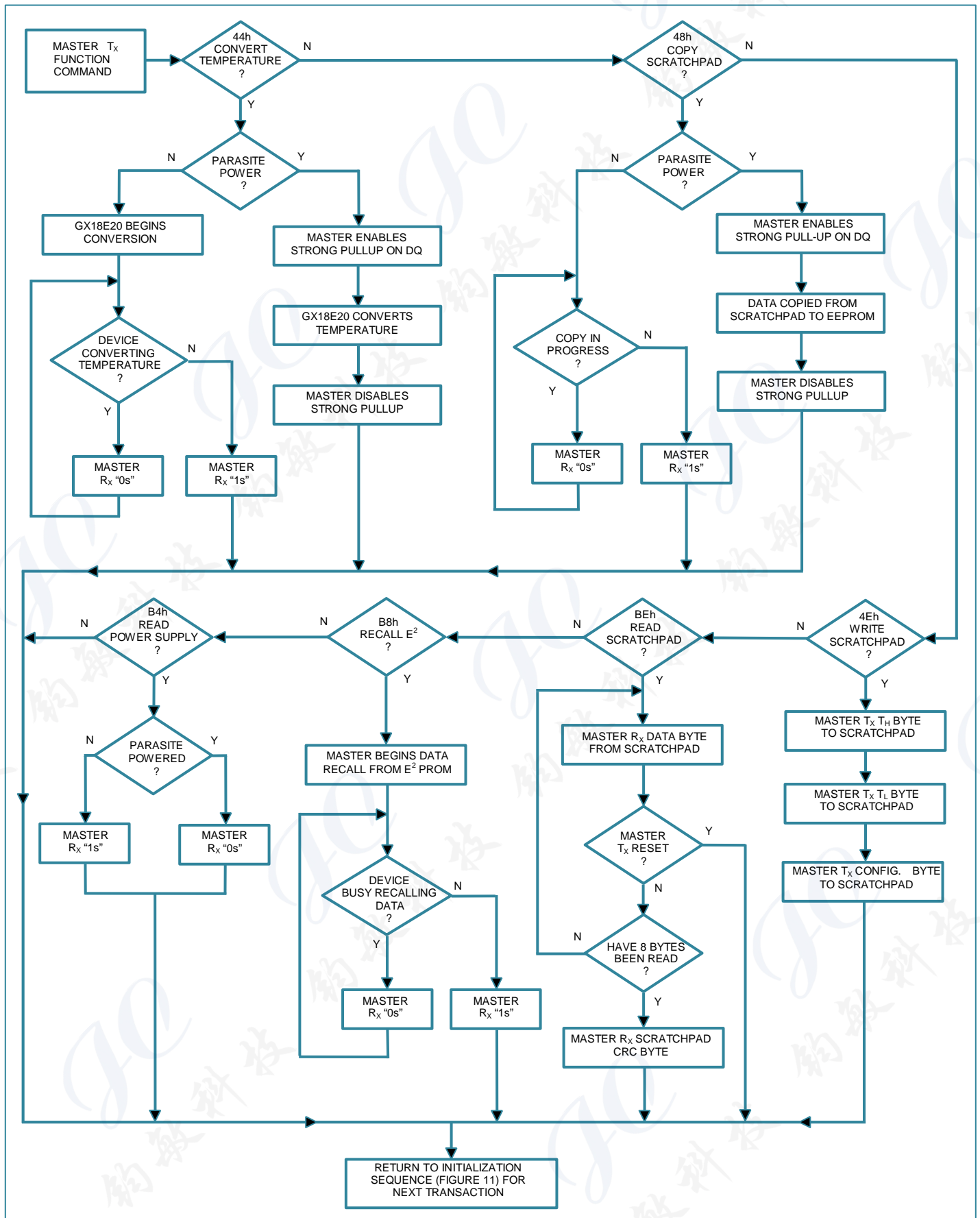
Figure 12. GX18E20 功能指令流程图
